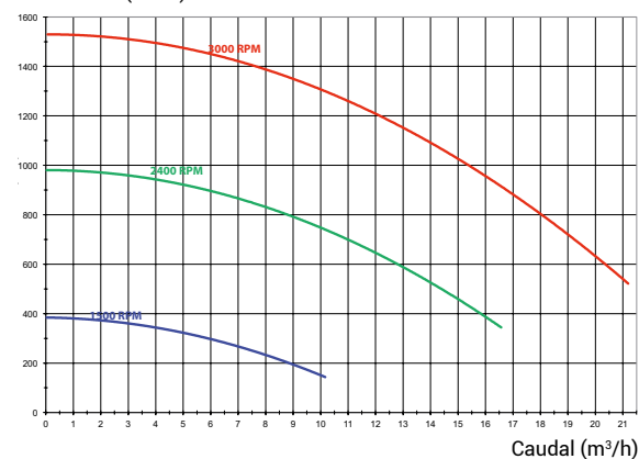
Curva del modelo 1,5 CV
