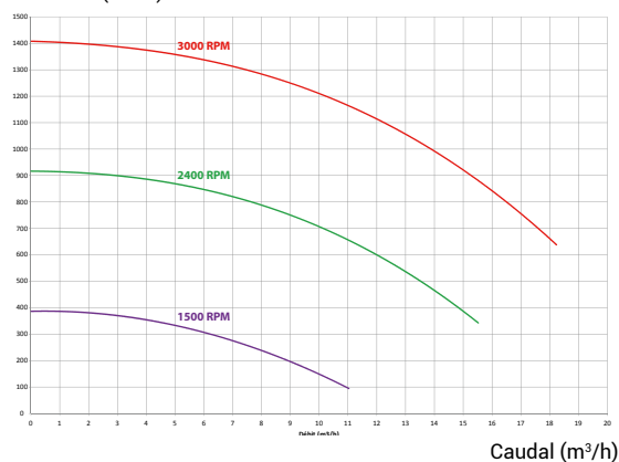
Curva del modelo 1 cv
