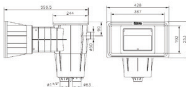
Dimensione Skimmer a inserti - bocca larga
