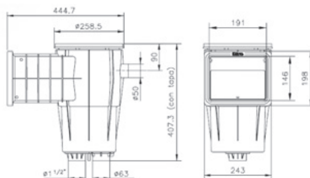
Dimensione Skimmer a inserti - bocca stretta
