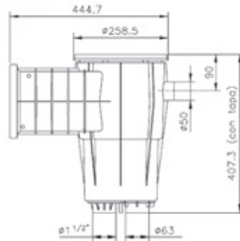
Maß - kleine Saugöffnung
