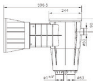
Maß - große Saugöffnung
