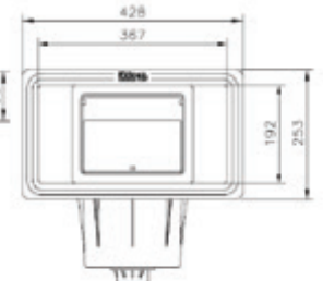
Maß - große Saugöffnung
