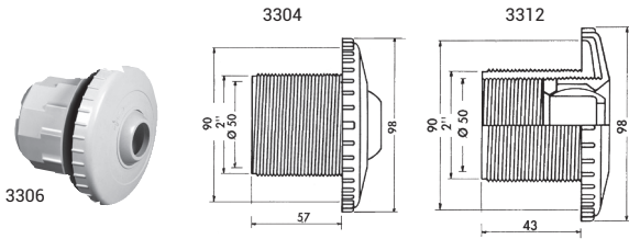
Buse de refoulement orientable 2" - 50 à coller pour piscine Béton et Coque
