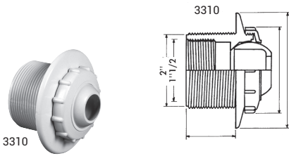
Buse de refoulement orientable 2" - 1 1/2" pour piscine Béton
