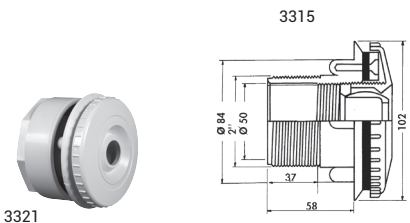
Buse de refoulement orientable 2" - 50 à coller pour piscines Liner et Panneaux
