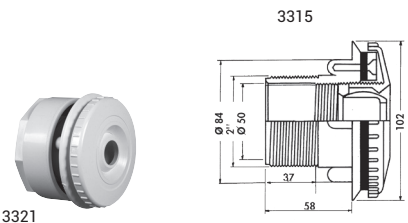
Boquilla de impulsión orientable 2" - 50 para encolar, para piscina Liner y Paneles
