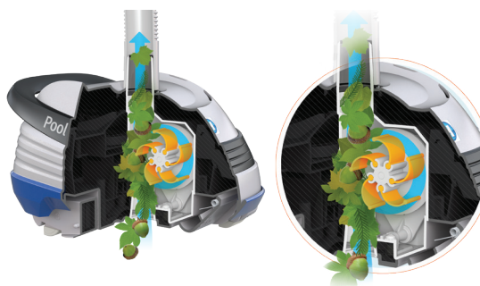
Tecnología patentada V-Flex®: turbina de álabes móviles para capturar los residuos grandes
