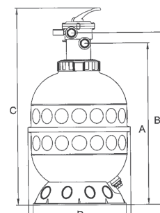
Dimensiones filtro HI Top
